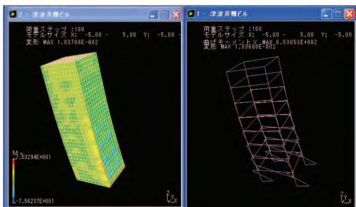
図2 TDAPIIIによる津波避難ビル計算例 左から変形+応力コンター図、変形+断面力図
