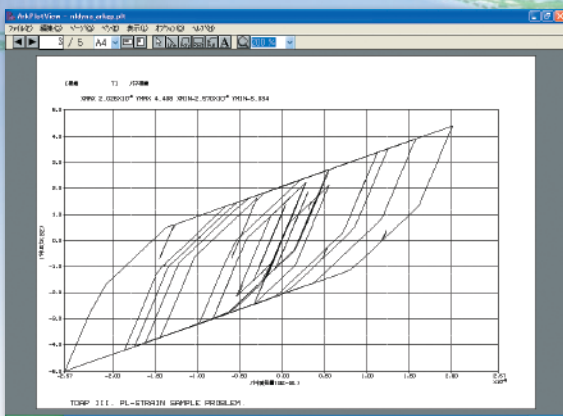
バネ履歴図
